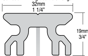
3853 Schiene für Nutstein-Montage
