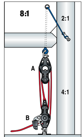
8:1 Kaskade: Das einfachste Cunningham besteht aus einer selbstklemmenden Talje am Mastfluss.
