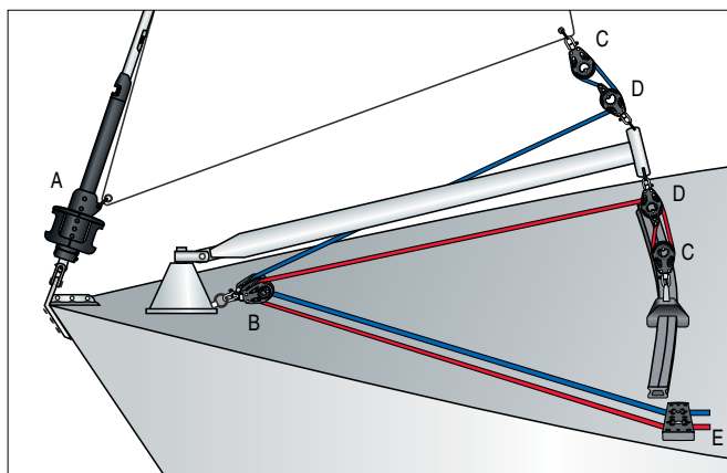
Selbstwender mit Fockbaum: Selbstwende-Fock und Stagsegel arbeiten bestens mit Roll-Reff System und Fockbaum. Zwei Schoten kontrollieren die Fock gegenüber dem Baum, bzw. den Baum.
