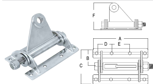
EINSTELLBARER BAUMBESCHLAG
